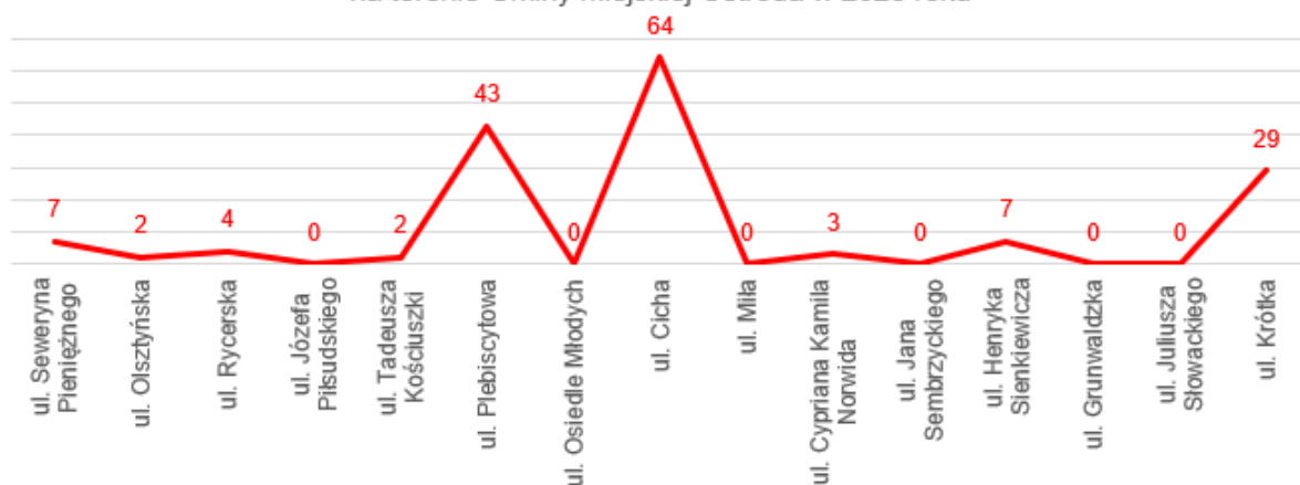
Liczba dni z PM10 powyżej poziomu 50 µg/m 3 na terenie Gminy Miejskiej Ostróda w 2023 roku
